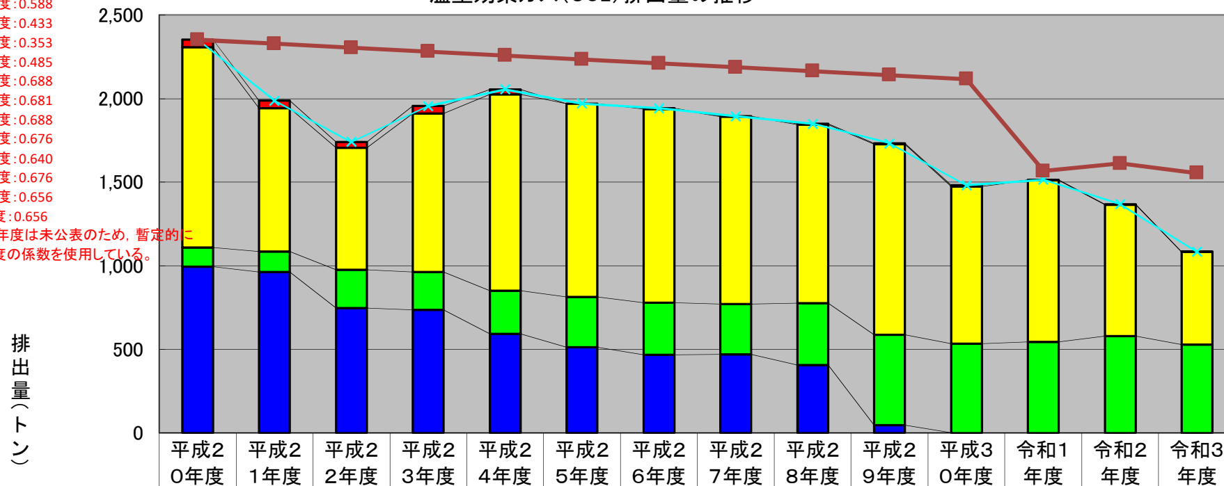
温室効果ガス(CO2)排出量の推移
