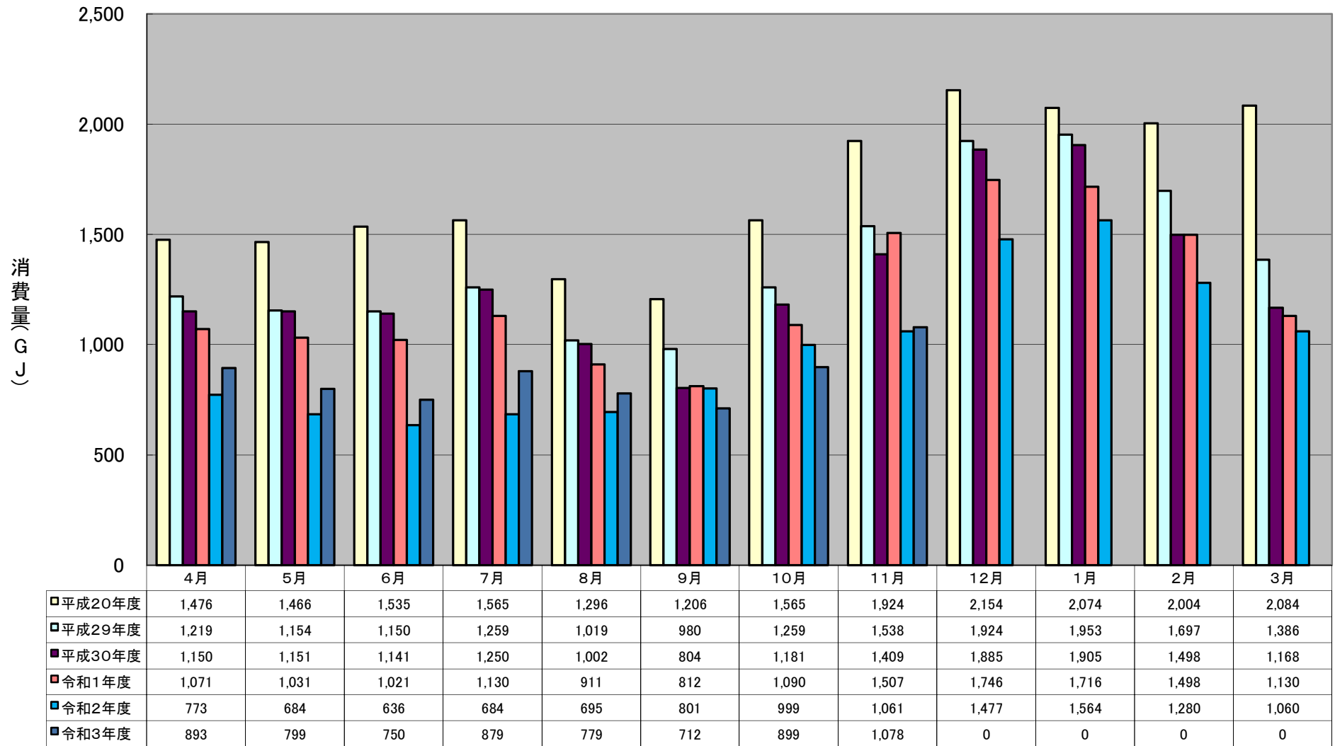
月別エネルギー消費量【電気】の推移（省エネ基準年平成20年度＋最近5年間）
