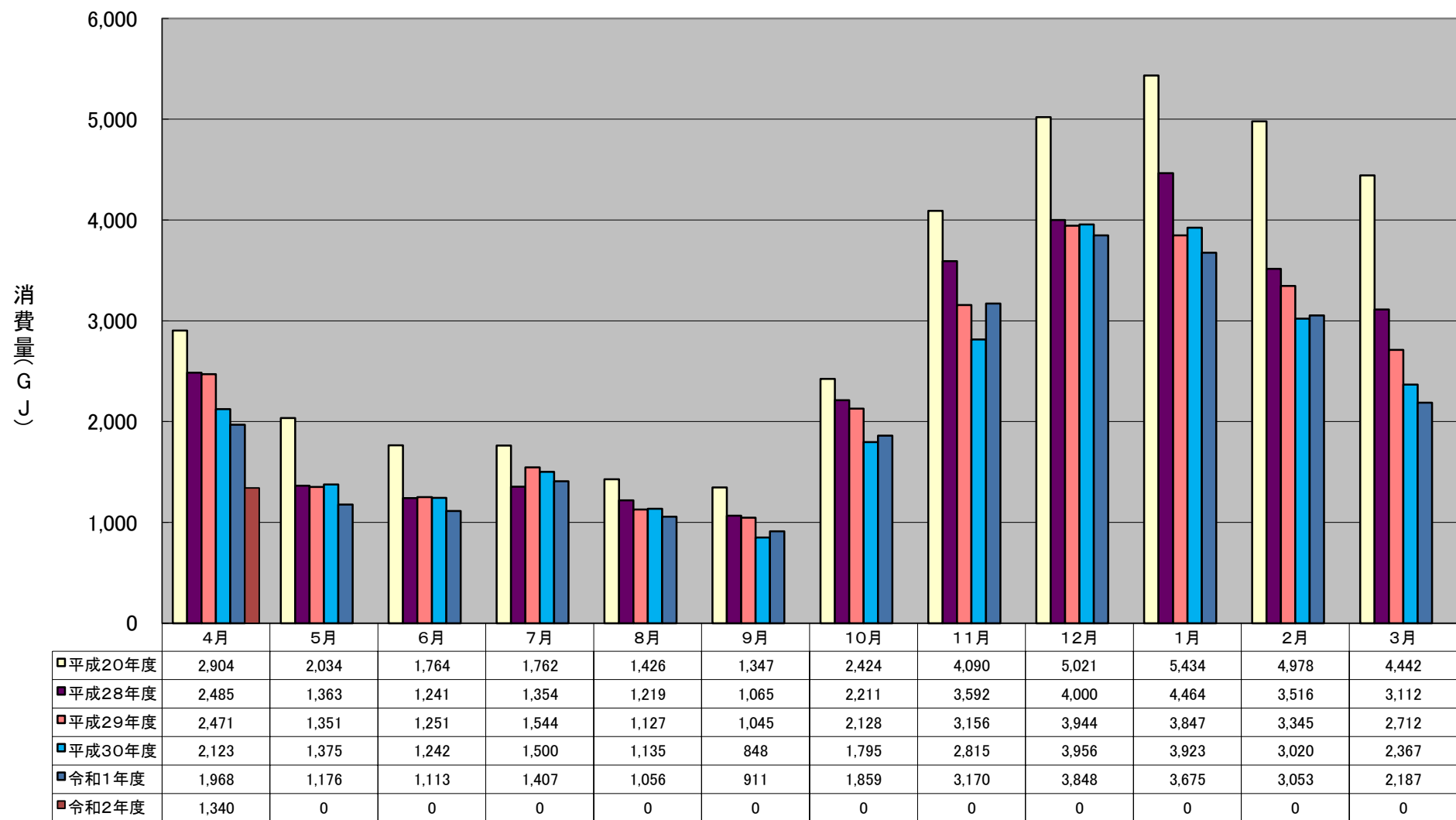
小樽商科大学全体のエネルギー消費量推移（省エネ基準年平成20年度＋最近5年間）
