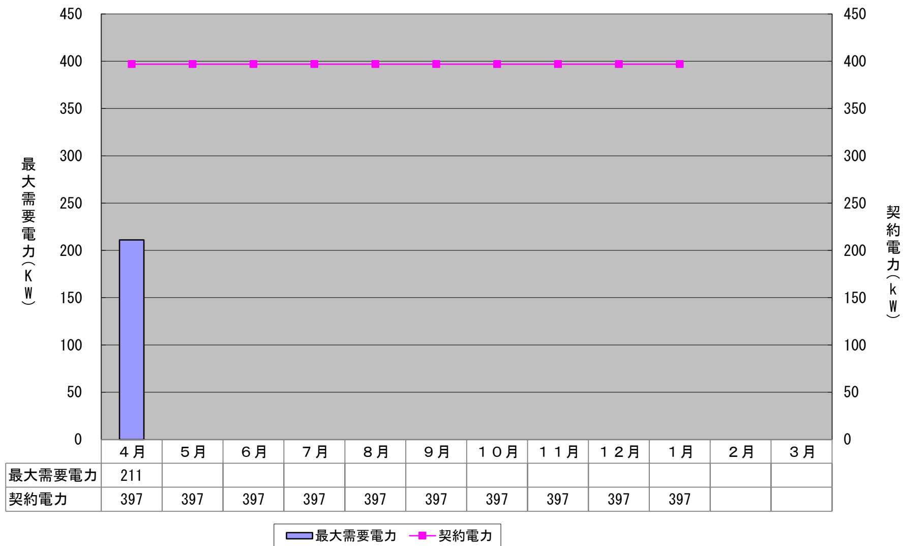
最大需要電力及び契約電力 （2020（令和2）年度）
