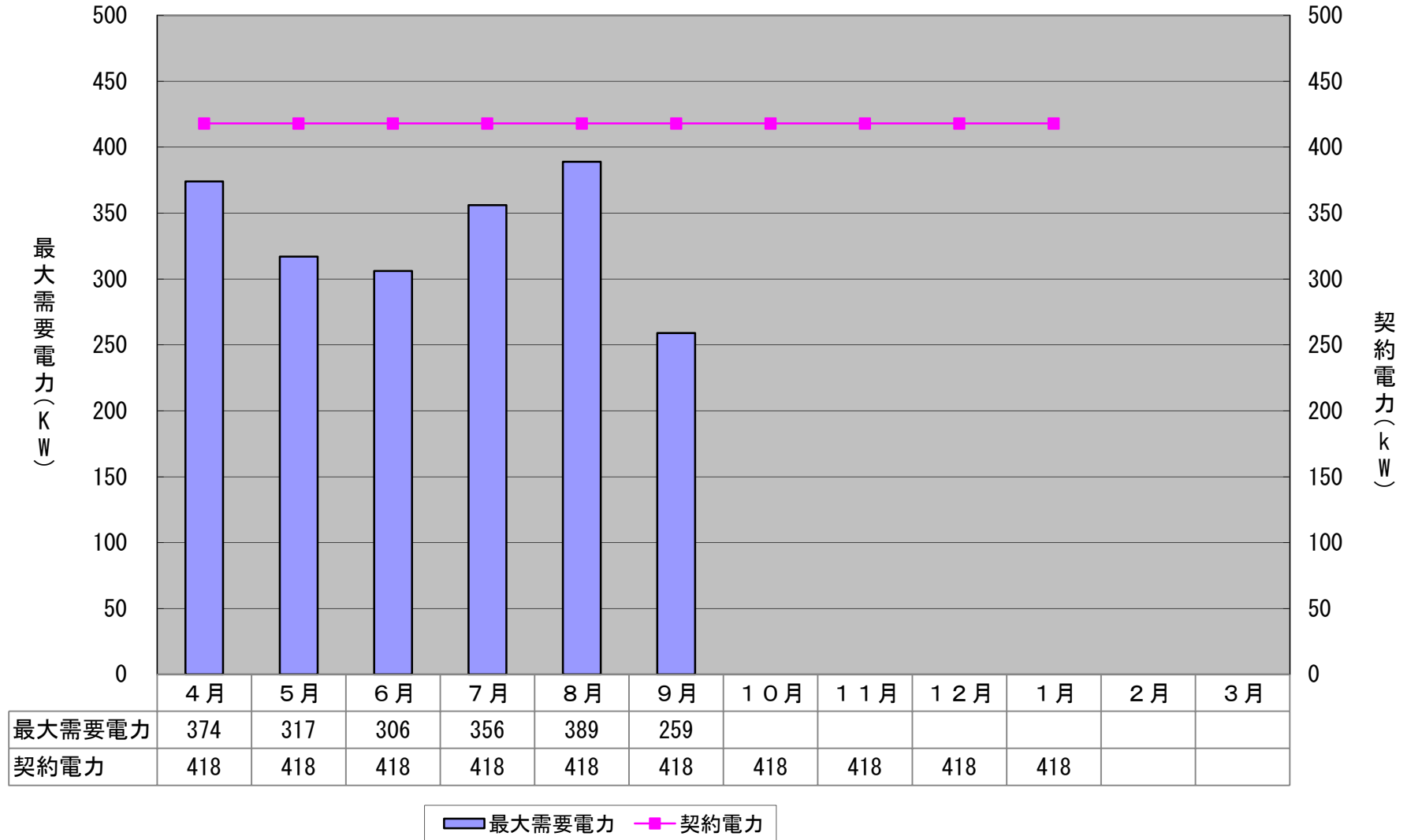
最大需要電力及び契約電力 (2019 (令和1) 年度)
