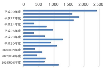
2号館GHP 7月消費量推移
