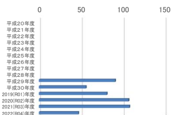
車庫ガス 10月消費量推移
